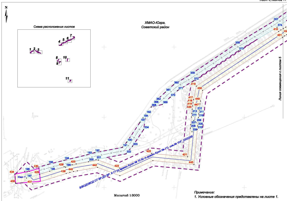
Лист 4, листов 11
