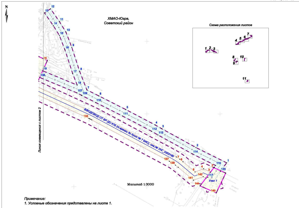
Лист 3, листов 11
