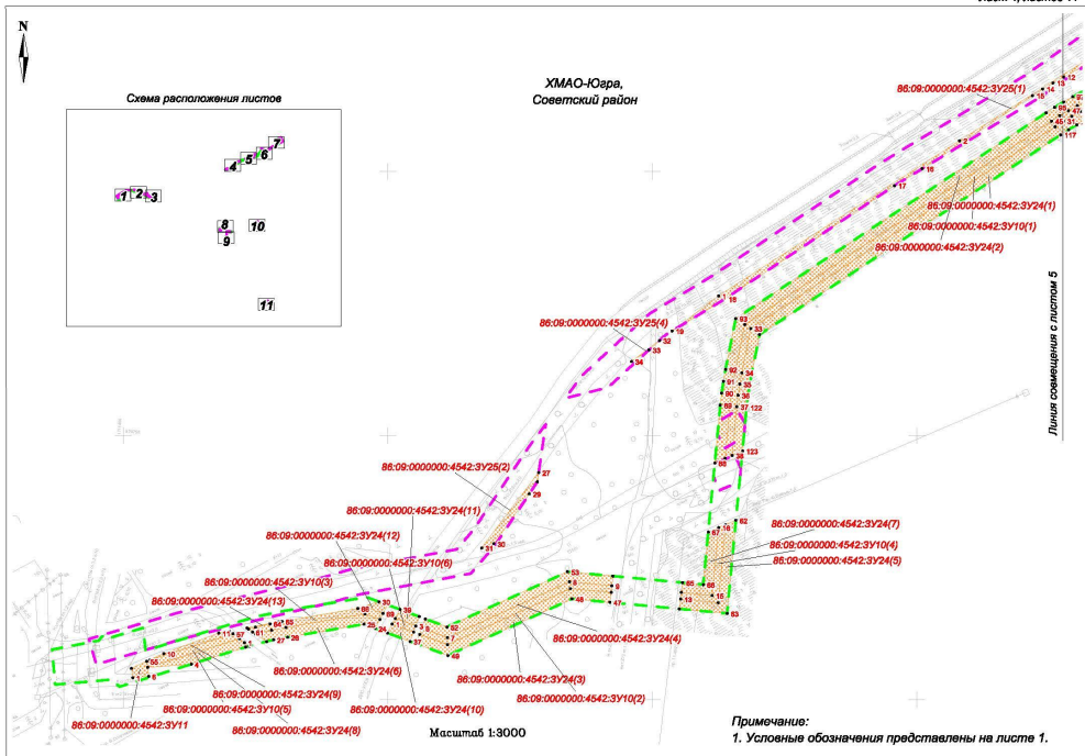
Лист 4, листов 11
