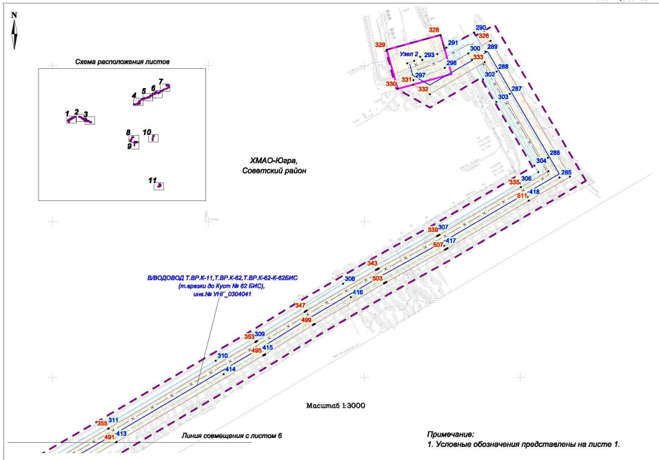
Лист 7, листов 11
